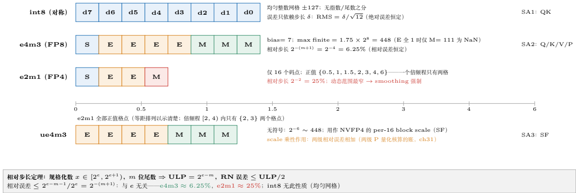
图 30.5: 四种量化格式的位域与值域对照 (int8 / e4m3 / e2m1 / ue4m3)。e4m3 的指数全 1 时仅 M=111 编码 NaN, 故满量程 448; e2m1 全部 16 个码点在数轴上标出, 直观呈现「一个倍频程内只有两格」。
