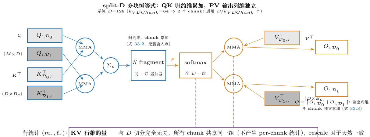
图 33.1: split-D 分块恒等式的数据流 (30.3.1 节)。QK 侧: D 是归约维, 各 chunk 的 Q_{:,D_c} K_{D_c,:}^\top 累加进同一个 S fragment (式 33.2, f32/s32 累加, 不引入新舍入点); PV 侧: D 是输出列维, 各 chunk 独立累加出 O_{:,D_c} 列段 (式 33.3), 无任何合并。softmax 的行统计 ( m_r, \ell_r ) 是 KV 行维的量——与 D 切分完全无关, 所有 chunk 共享同一组 (灰色 = chunk 身份, 两图同语义)。
