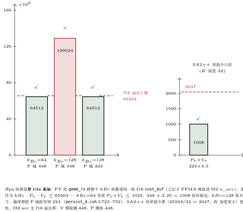
图 32.1: f16 PV 累加器的整 tile 域预算 (式 32.4)。条形为 kBc \times P_r \times V_r : kBc=64 与「 kBc=128 + P 域自动收窄到 224」都恰为 64512, 贴住 65504 上限; kBc=128 且 P 仍 448 则 129024 约 2 倍超限。右: SA2++ 按单条 MMA ( K=32 ) 核算的界 2047 更松 ( P_r=224, V_r=4.5 双侧收窄)。f32 acc 路径无此约束。
