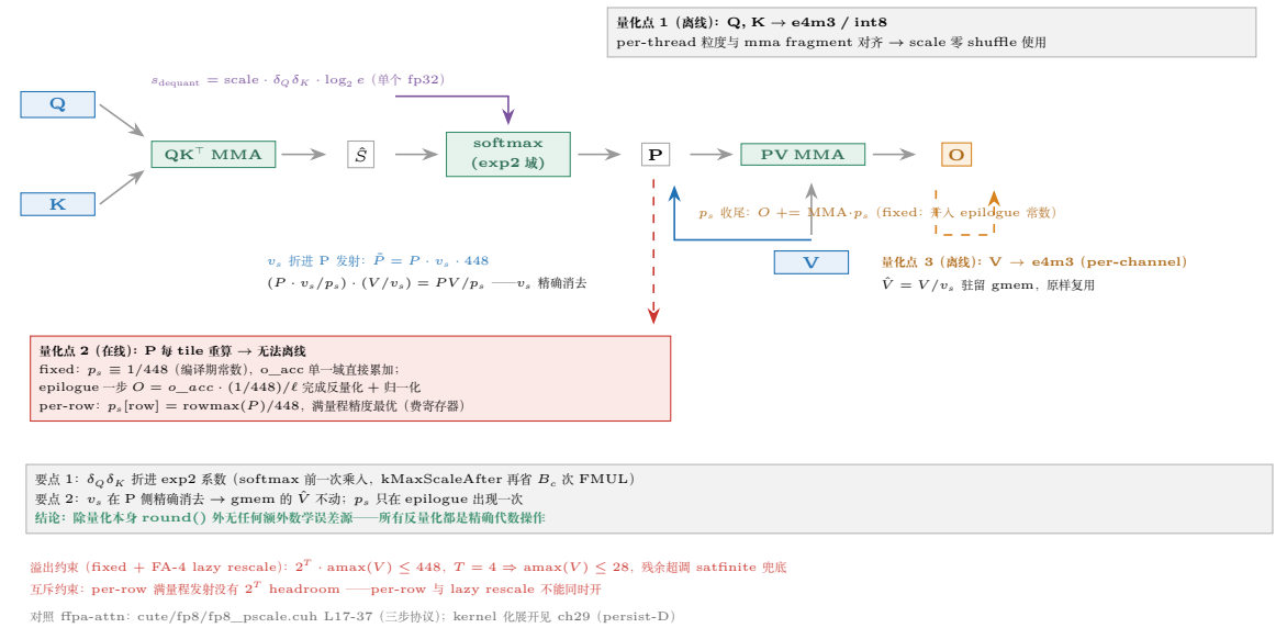
图 30.6: attention 的三个量化点与 scale 流向: \delta_Q \delta_K 折进 exp2 系数 (式 30.4)、 v_s 在 P 侧精确消去 (式 30.5)、 p_{scale} 在 epilogue 一步收尾。
