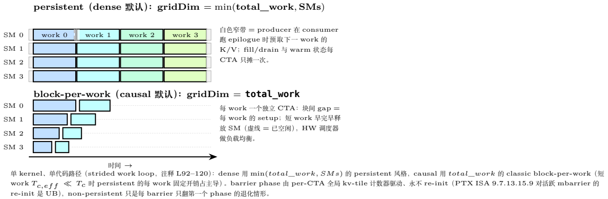
图 35.1: dense persistent 与 causal block-per-work 的 grid 调度对比 (同一 kernel、同一代码路径, runtime grid 定风格)。上: \min(\text{total\_work}, \text{SMs}) 个 CTA 按 strided work loop 认领, fill/drain 每 CTA 摊一次, producer 在 epilogue 期间预取下一 work 的 K/V; 下: 每 work 一个 CTA, 短 work 早完早释放 SM。
