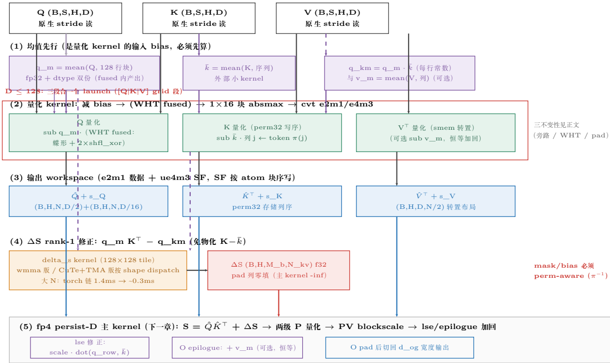
图 34.6: fp4 前处理链数据流 ( D \leq 128 走 fused 单 launch 路径): \bar{k}/q_m 均值先行的原因是它们是量化 kernel 的输入 bias; hadamard 下 q_m^{rot} 在 fused kernel 内顺带产出。
