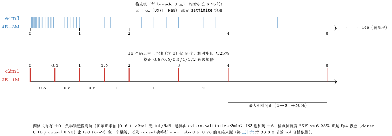
图 34.1: e2m1 vs e4m3 的格点数轴 (同一 [0, 6] 区间)。上: e4m3 每个 binade 8 个格点、相对步长 6.25%, 满量程 \pm 448 ; 下: e2m1 正半轴全部格点仅 \{0, 0.5, 1, 1.5, 2, 3, 4, 6\} 、相对步长约 25%, [4, 6] 段相对间距最大 (+50%)。fp4 的容差天然比 fp8 宽一个量级的格式层根源。
