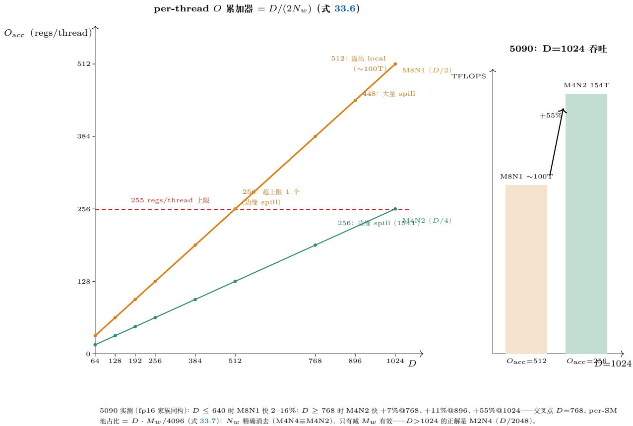
图 33.2: 寄存器墙的定量视图。左: per-thread O 累加器 = D/(2N_w) (式 33.6) ——M8N1 的 D/2 在 D=512 达 256 (超 255 上限 1 个, 边缘 spill)、 D \geq 896 大量 spill、 D=1024 溢出 local memory (~100T); M4N2 的 D/4 同点仅 256 (154T)。右: 5090 实测 D=1024 吞吐对比 (+55%)。下: per-SM 池占比 D \cdot M_w / 4096 (式 33.7) 中 N_w 精确消去——加 N-warp 不降总量, D > 1024 只能走 M2N4。
