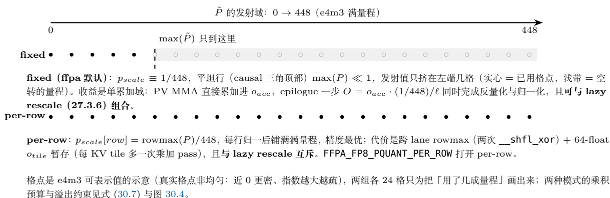
图 30.2: fixed 与 per-row 两种 p_{scale} 策略的发射域利用率 (27.3.5 节)。上: fixed 的 p_{scale} \equiv 1/448 是编译期常数, 平坦行的 \max(P) \ll 1 使发射值只占量程左端一小段, 其余量程空转——换来的是单累加域与「可与 lazy rescale 组合」; 下: per-row 用 \text{rowmax}(P)/448 把每一行拉满, 精度最优, 代价是跨 lane rowmax 归约与 64-float 的 o_{tile} 暂存, 且与 lazy rescale 互斥。
