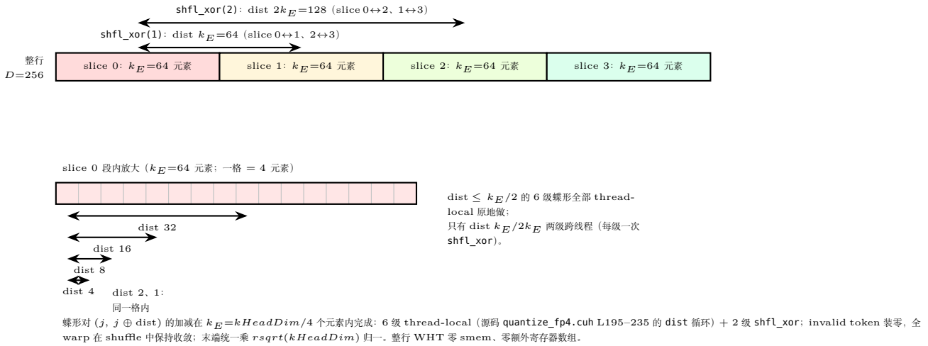
图 34.4: fused WHT 的蝶形距离分层 ( D=256 , 4 线程一 token、每线程 k_E=64 连续元素)。距离 < k_E 的 6 级蝶形全在 thread-local 数组内; dist k_E 与 2k_E 两级各用一次 shfl_xor(1)/shfl_xor(2) 跨 slice 交换——零 smem、零额外寄存器数组。
