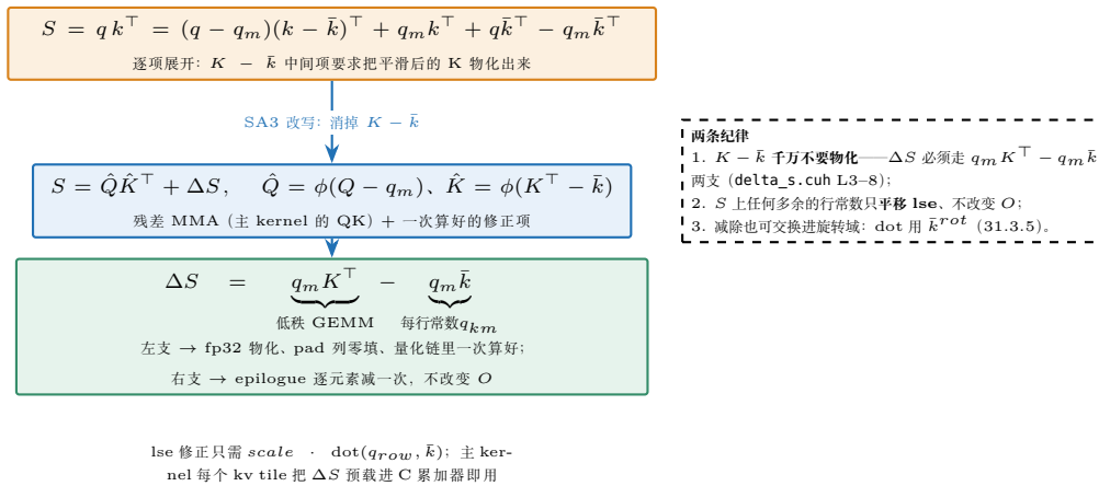
图 34.2: \Delta S 的 rank-1 恒等式。四项展开折叠为「残差 MMA + 修正项」: \Delta S 由低秩 GEMM q_m K^T 与每行常数 q_m \bar{k} 两支等价构成, K - \bar{k} 永不物化; 行常数只平移 lse。
