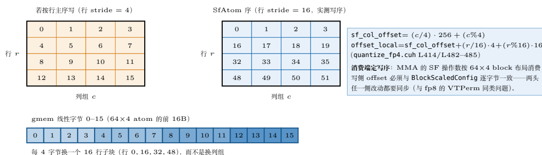
图 34.3: SF 字节的写序由消费端决定 ( V^T 量化链)。同一 (r, c) 单元格在行主序假设下偏移 4r + c ，在 SfAtom 序下偏移 16r + c ：每 4 个列组构成 64 \times 4 的 256B atom，atom 内按 16 行子块交错。写侧 (sf_col_offset/offset_local) 与 MMA 的 BlockScaledConfig 必须逐字节一致。
