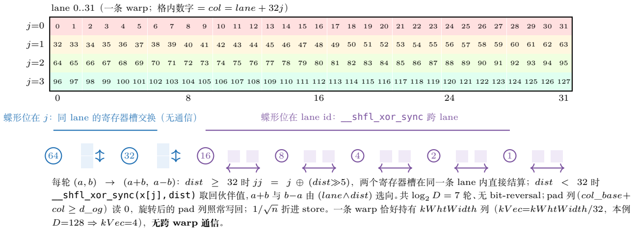
图 31.4: radix-2 蝶形的距离二分 (hadamard.cuh L40-92, 本例 D=128 、 kWhWidth=D )。上：列归属—— j 是寄存器槽、lane 是 warp 内线程，格内数字 col = lane + 32j 满足索引律，右下角 127 = size - 1 ；一条 warp 覆盖整行 128 列。下：七轮的「距离阶梯」—— dist \geq 32 的 bit 落在 j 上（同 lane 两个寄存器槽直接加减，无通信）， dist < 32 的 bit 落在 lane id 上（ __shfl_xor_sync 跨 lane）；每轮一个 bit， 1/\sqrt{n} 折进 store。
