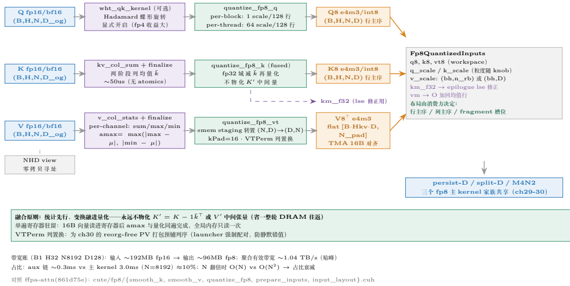
图 31.5: fp8 前处理链全景: 三泳道 (Q/K/V) 各自的统计 \rightarrow 变换 \rightarrow 量化 kernel 与输出 workspace 布局。smoothing 与量化融合在同一 kernel 内 (无中间落盘); V^T 的列 pad 兼顾 TMA 16B 对齐与置换写。
