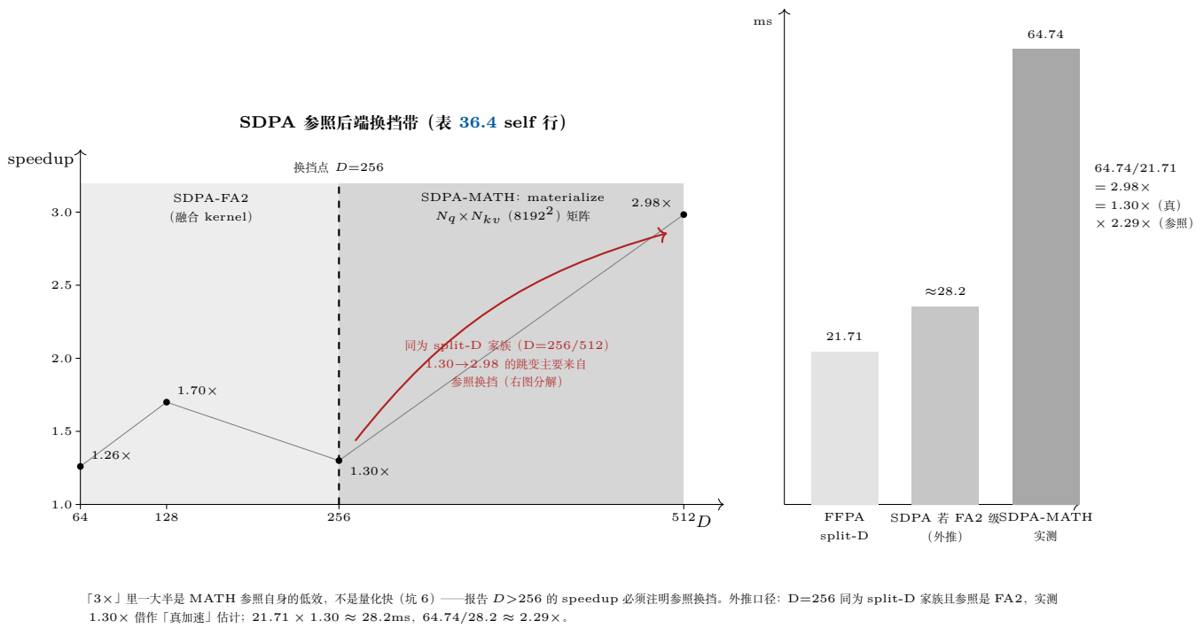
图 36.1: 参照系视角看表 36.4 的 self 行。左: SDPA 参照随 D 换挡——FA2 只覆盖 D \leq 256 , 更大 D 静默落到 MATH (materialize N_q \times N_{kv} 矩阵); 四个 speedup 点 (1.26/1.70/1.30/2.98×) 落在换挡带上, D=512 的跳变与 kernel 无关。右: D=512 的 2.98× 归因——以 D=256 同家族 (split-D、FA2 参照) 实测 1.30× 为真加速估计, MATH 参照自身再慢 \times 2.29 : 「3×」的大头是参照低效 (坑 6)。
