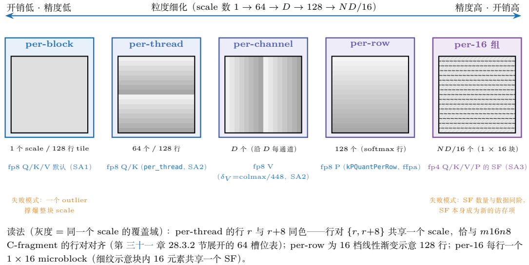
图 30.1: 量化粒度谱系五联网络 (表 30.2 的可视化, 缩略网格为 16 行 \times 16 列)。从左到右: per-block 整块共享 1 个 scale; per-thread 按 C-fragment 行对 \{r, r+8\} 分档 (128 行块共 8 \times 8 = 64 个, 零 shuffle 消费); per-channel 沿 D 每通道一个; per-row 每 softmax 行一个 (128 个); per-16 每行一个 1 \times 16 microblock (NVFP4 的 SF)。顶部双向轴是整条谱系的 trade-off: 粒度越细精度越高, 但 scale 的存储、传递与消去开销同步上涨, 且必须与 MMA 的 fragment 布局对齐——谱系两端的失败模式分别是对 outlier 的脆弱性与 SF 自身的访存账。
