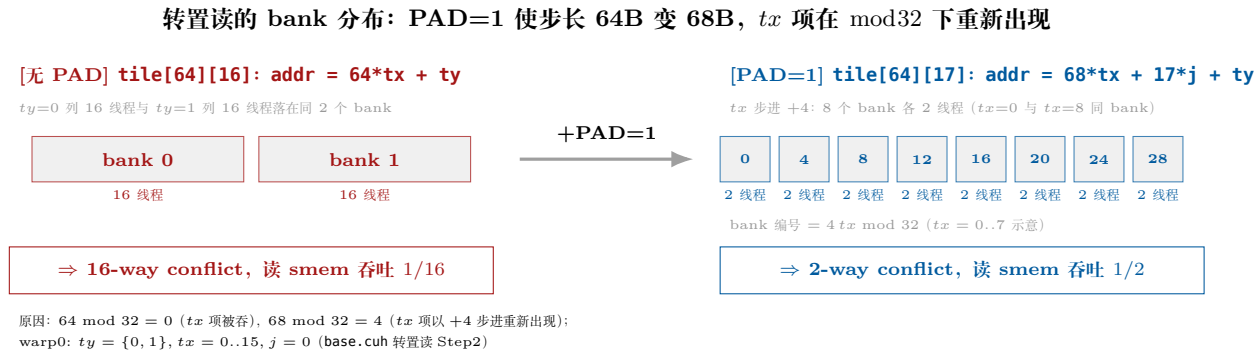
图 8.5: bank conflict vs padding—PAD=1 使步长 64B 变为 68B, tx 项在 mod 32 下重新出现, 16-way 冲突降为 2-way (读 smem 吞吐 1/16 \rightarrow 1/2 )。
