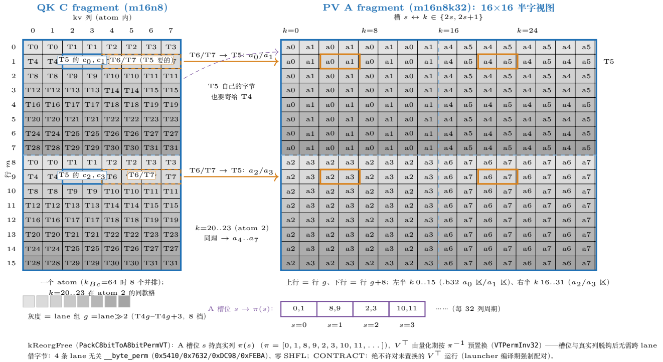
图 32.2: C→A fragment 的 lane→值映射 (reg2reg_8b.cuh L14–34 头注释的网格化)。左: QK C fragment (m16n8), 每 lane 4 值 c_0-c_3 落在行 g/g+8 的列对 \{2t, 2t+1\} ; 右: PV A fragment (m16n8k32) 的 16×16 半字视图, 格值 a_0-a_7 为 e4m3x2 半字寄存器, 四象限对应源码.b32 a_0-a_3 ; 两面板灰度同语义 (lane 组 g = \text{lane} \gg 2 , 8 档)。中: t=1 (T5) 的自然 A 需要 k \in \{4..7\} \cup \{20..23\} (行 g 与 g+8 ), 在 C 视图里属 T6/T7——纯 lane 内置换凑不齐, 即 16 SHFL + 32 PRMT (ReorgC8bitToA8bit) 的根源。下: kReorgFree 的出路——槽位持 \pi(s) 、 V^\top 预置换, 4 条 lane 无关 __byte_perm、零 SHFL。
