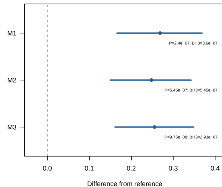
binary AUC
