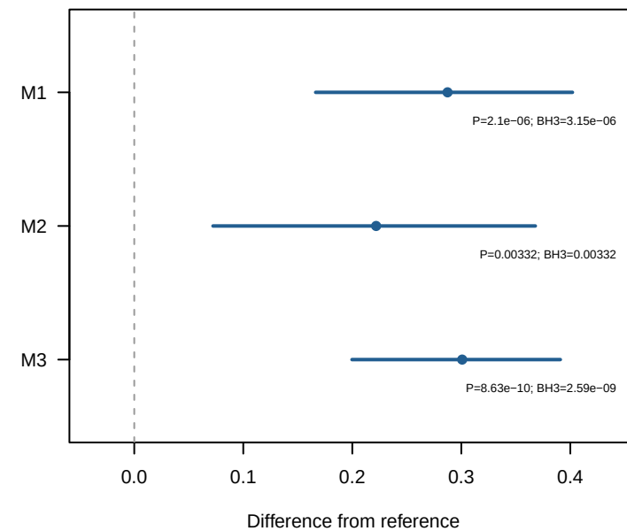
binary AUC
