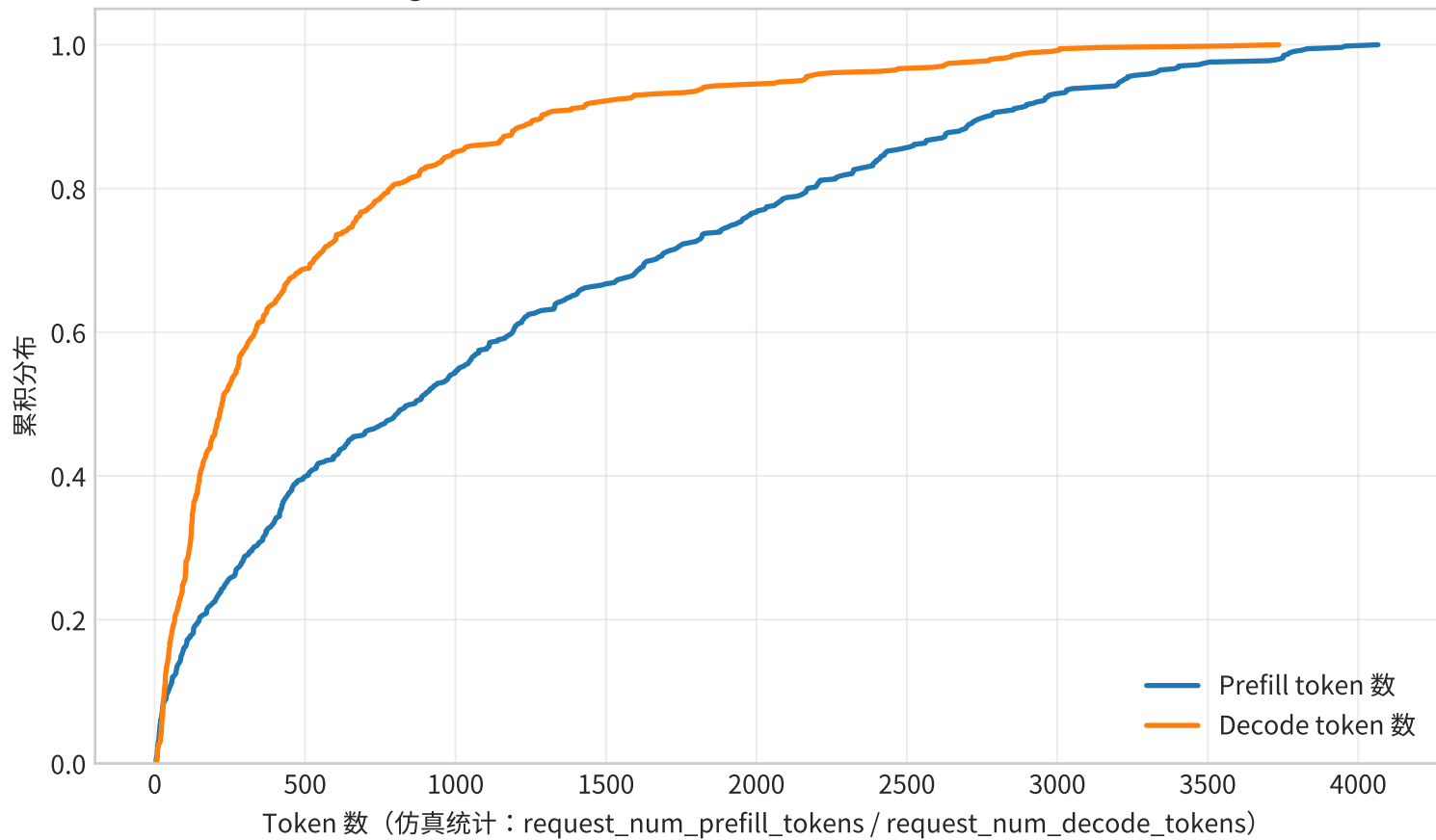
Code Agent Trace : Prefill 与 Decode token 长度累积分布 (CSV)
