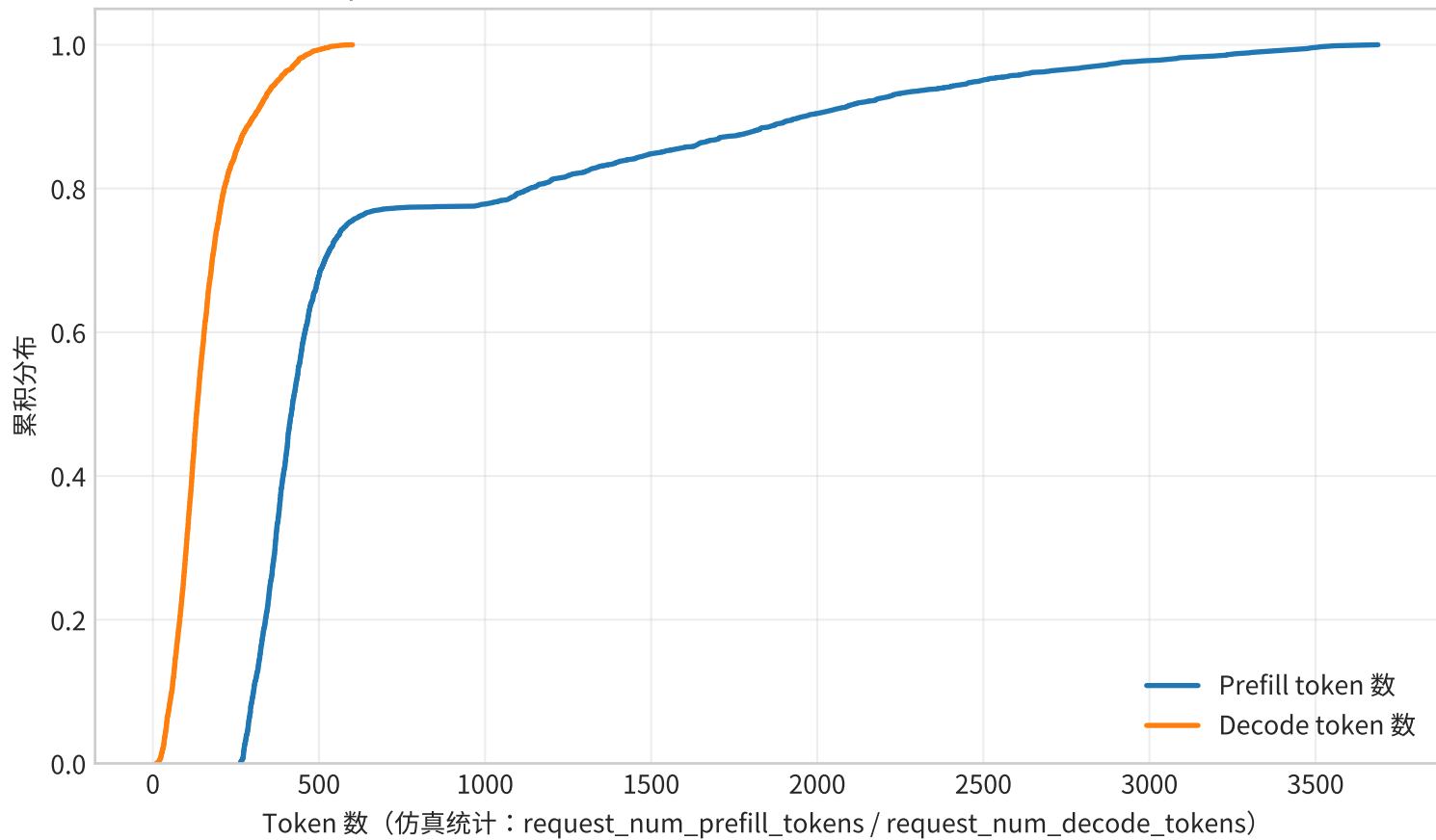
MapReduce Trace：Prefill 与 Decode token 长度累积分布（CSV）
