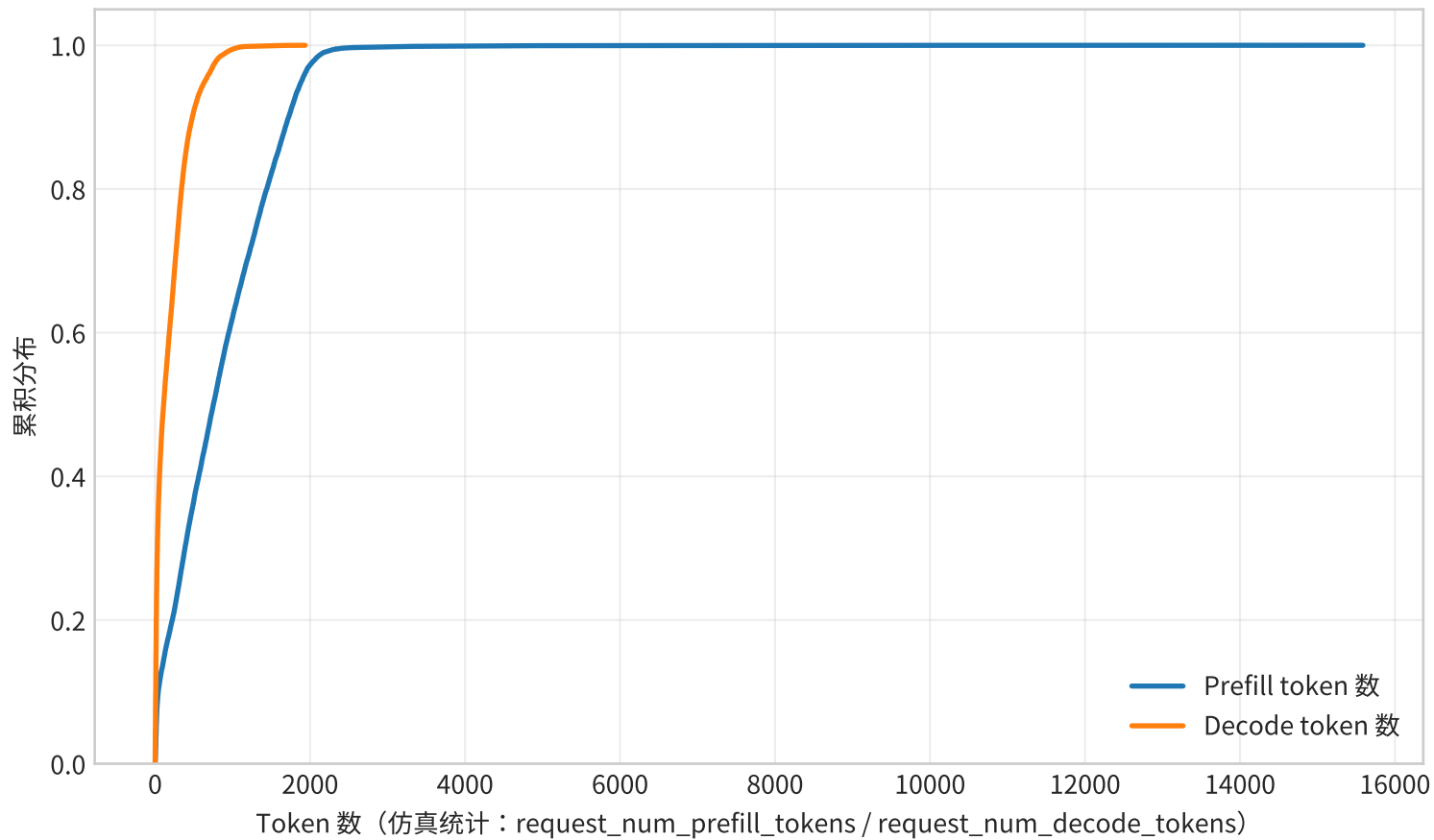
ShareGPT V3 : Prefill 与 Decode token 长度累积分布 (CSV)
