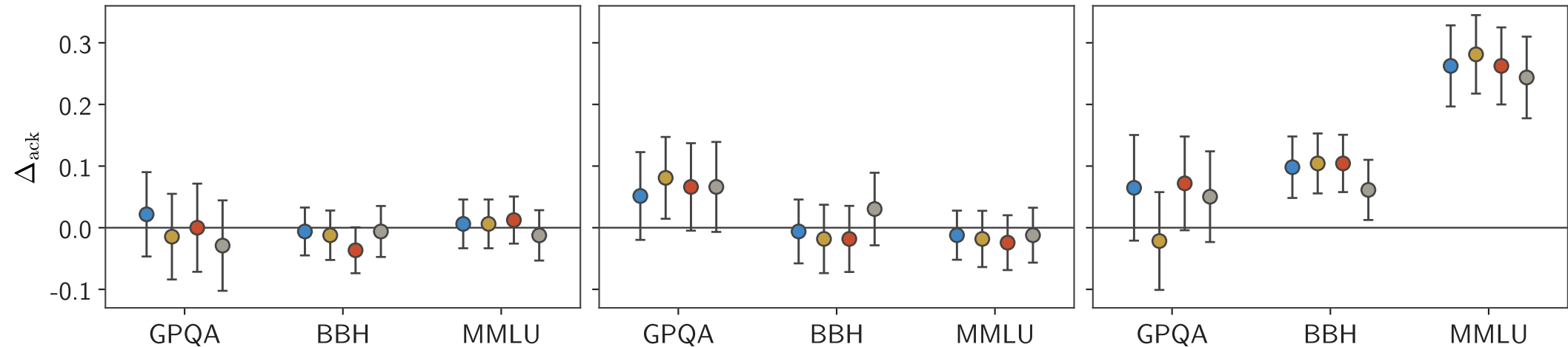
Gemma-3 4B
