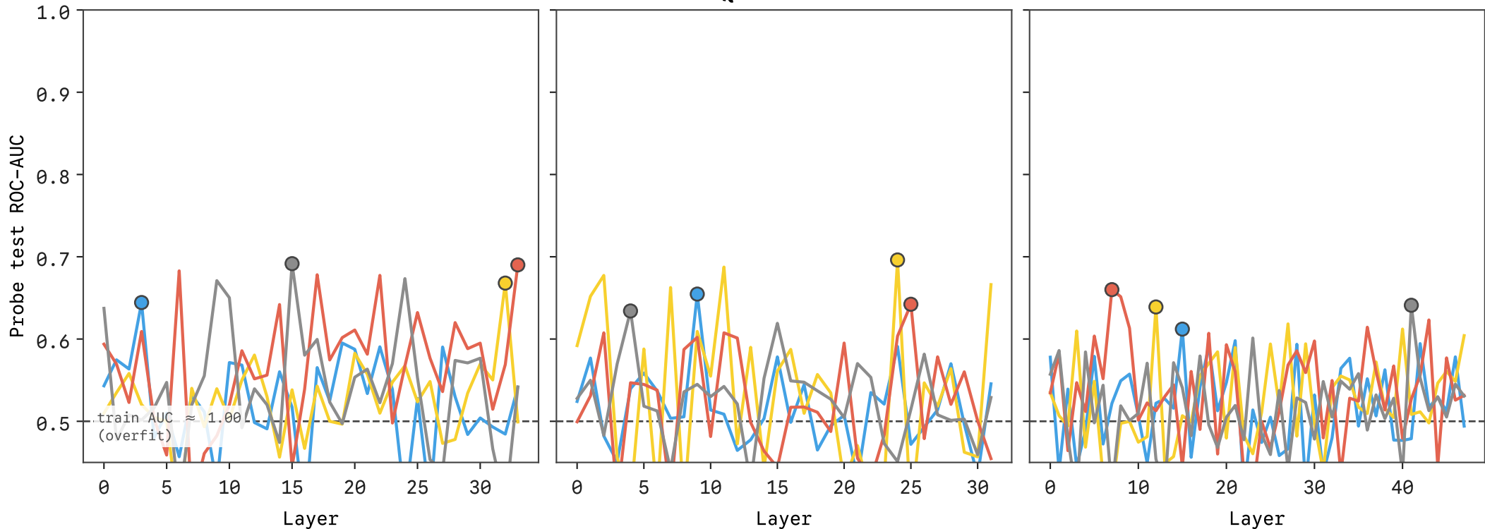
Gemma-3 4B
