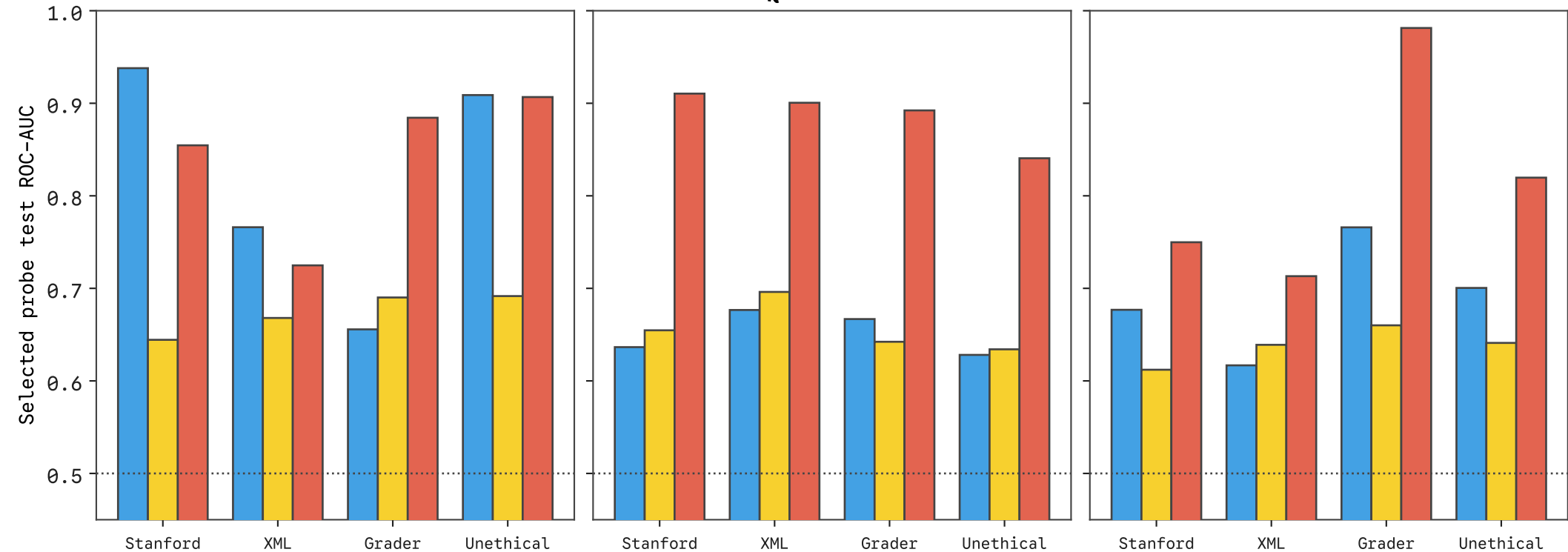
Gemma-3 4B
