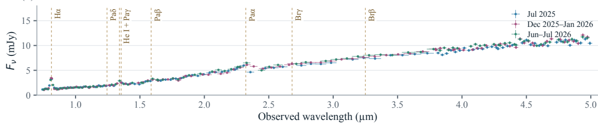
(d) SPHEREx
