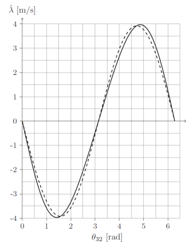
FIGURE 1.3 – Évolution théorique (—) et approximée (- -) de la vitesse \dot{\lambda} pour \dot{\theta}_{32} = 3000 \text{ tr min}^{-1} .
