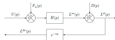
FIGURE 5 – Modèle du procédé pour la conception de la loi de commande de la chaîne d'asservissement
