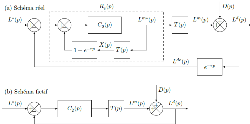
FIGURE 8 – Modèle de commande avec une boucle interne intégrée
