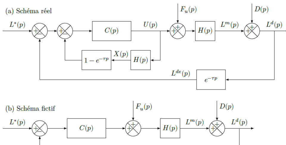
FIGURE 7 – Structure de commande adaptée aux systèmes à retard
