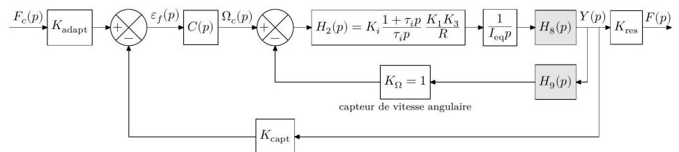
FIGURE 1.16 – Schéma-blocs de l'asservissement de la force développée par un actionneur linéaire
