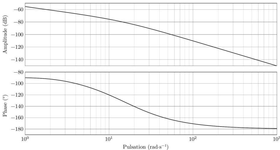
FIGURE 1.18 – Diagramme de Bode de H_{BO f}(p)
