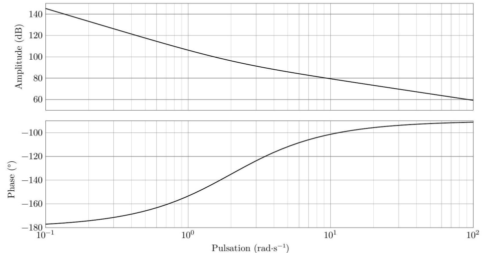
FIGURE 1.15 – Diagramme de Bode de H_{BOv}(p)
