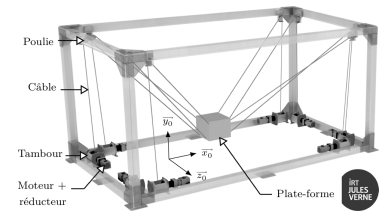
FIGURE 1.11 – Robot à câbles CAROCA
