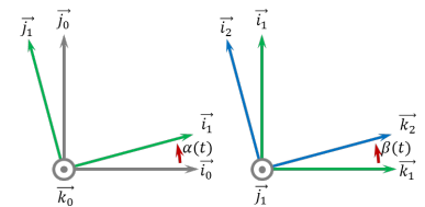
FIGURE 5.4 – Paramétrage
