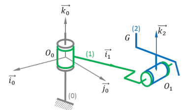
FIGURE 5.3 – Modélisation cinématique
