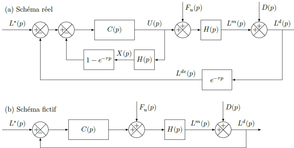
FIGURE 12.5 – Structure de commande adaptée aux systèmes à retard
