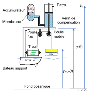
FIGURE 1.13 – Schéma d'implantation du PHV (non à l'échelle)
