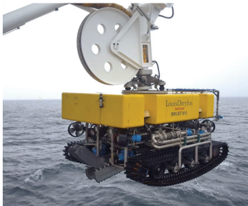
FIGURE 1.11 – ROV suspendu à la grue portique
