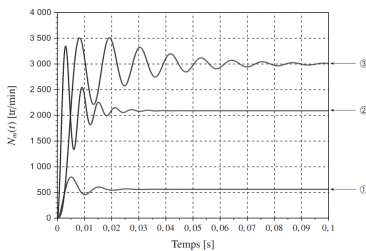
FIGURE 1.8 – Évolutions simulées de \omega_m(t) .
