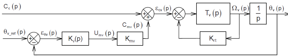
FIGURE 1.17 – Schéma-blocs de l'unité de pilotage avec retour tachymétrique
