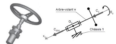
FIGURE 1.13 – Unité de pilotage (chaîne d'énergie) et schéma cinématique
