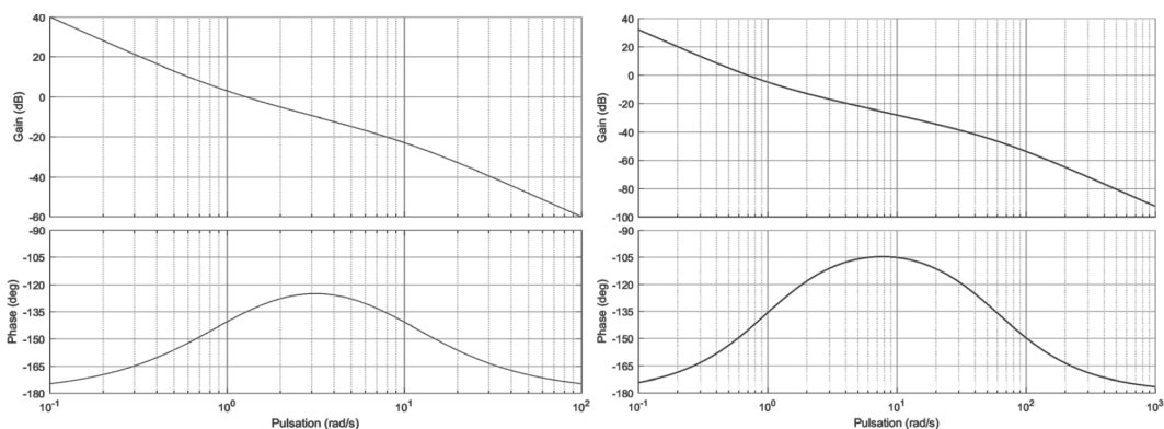
FIGURE 1.11 – Lieux de transfert de FTBO_{v1}(p) et FTBO_{v2}(p)
