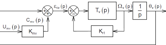
FIGURE 1.8 – Schéma-blocs de l'unité de pilotage avec retour tachymétrique
