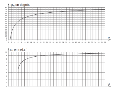
FIGURE 1.15 – Abaques de réglage de H(p) en fréquentiel
