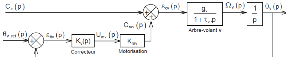
FIGURE 1.5 – Schéma-blocs de l'unité de pilotage
