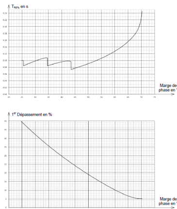
FIGURE 1.9 – Abaques de réglage en temporel de l'unité de pilotage corrigée avec retour tachymétrique
