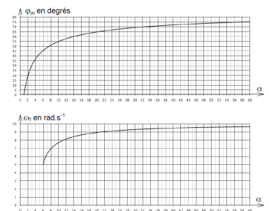
FIGURE 1.6 – Abaques de réglage de H(p) en fréquentiel
