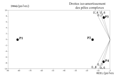
FIGURE 1.2 – Carte des pôles
