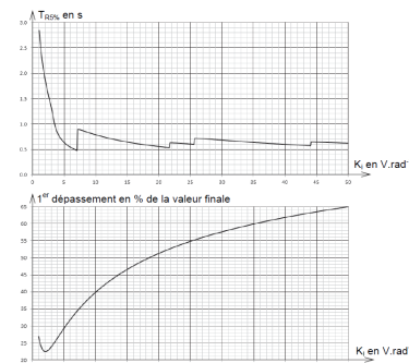
FIGURE 1.7 – Abaques de réglage en temporel de l'unité de pilotage corrigée
