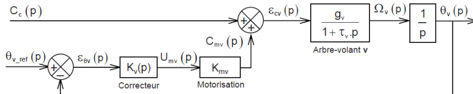
FIGURE 1.14 – Schéma-blocs de l'unité de pilotage
