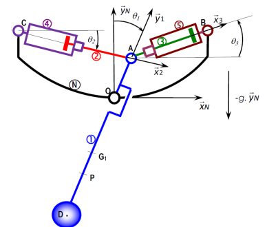
FIGURE 3 – Modèle 2D
