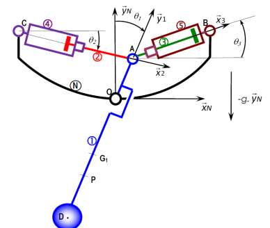
FIGURE 7 – Modèle 2D
