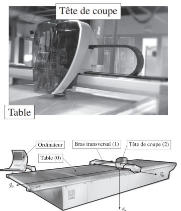
FIGURE 1 – Structure d'une table de découpe de tissus
