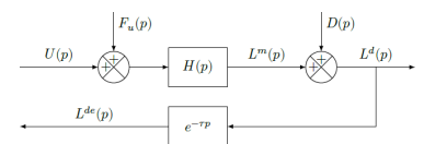
FIGURE 11.4 – Modèle du procédé pour la conception de la loi de commande de la chaîne d'asservissement
