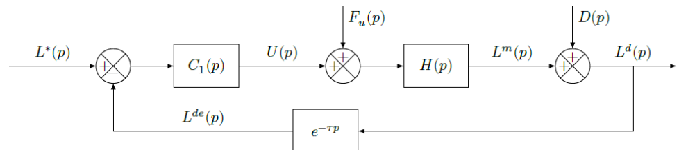
FIGURE 11.5 – Structure de commande à une boucle
