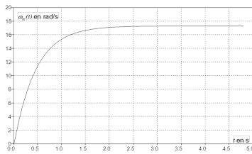
FIGURE 11.10 – Réponse en vitesse à un échelon de tension u(t) d'amplitude 100 V.
