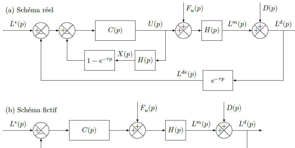
FIGURE 11.6 – Structure de commande adaptée aux systèmes à retard
