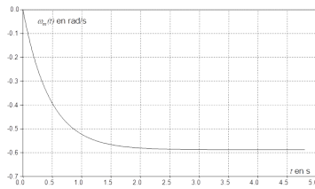
FIGURE 11.15 – Réponse en vitesse à un échelon de couple de perturbation c_r(t) d'amplitude 1000 N m.
