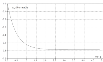
FIGURE 11.11 – Réponse en vitesse à un échelon de couple de perturbation c_r(t) d'amplitude 1000 N m.
