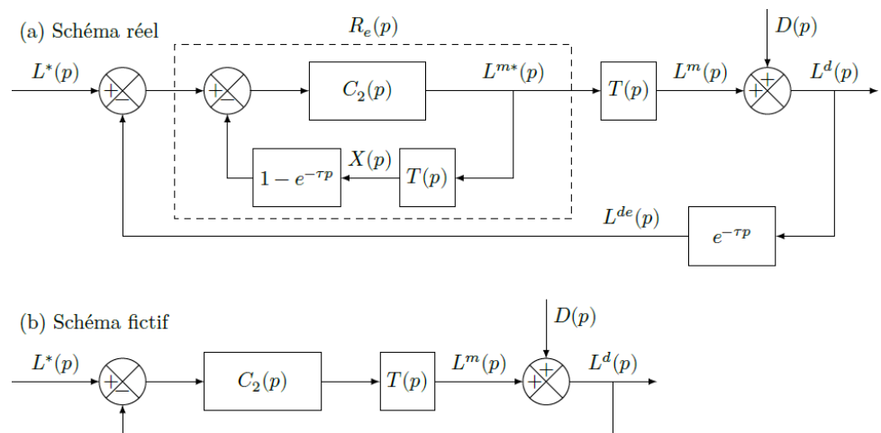
FIGURE 11.7 – Modèle de commande avec une boucle interne intégrée
