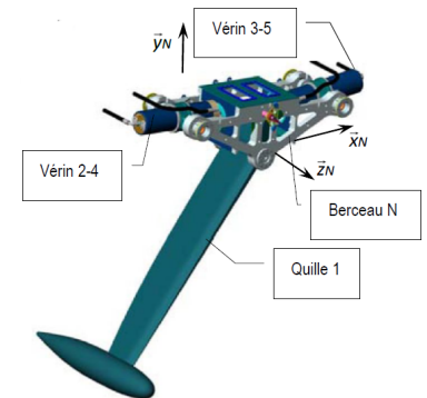
FIGURE 11.9 – Modèle volumique 3D
