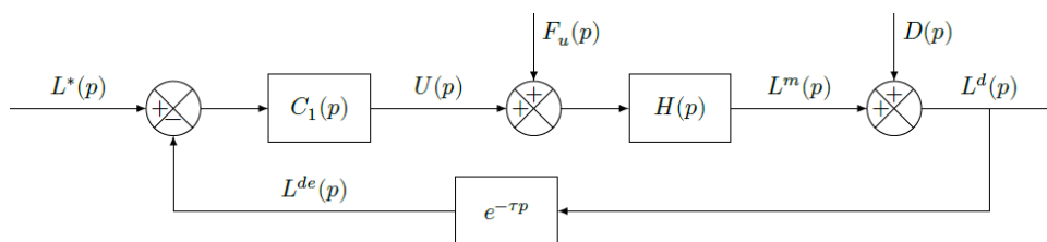
FIGURE 12.4 – Structure de commande à une boucle
