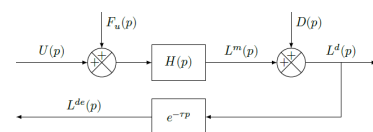
FIGURE 12.3 – Modèle du procédé pour la conception de la loi de commande de la chaîne d'asservissement
