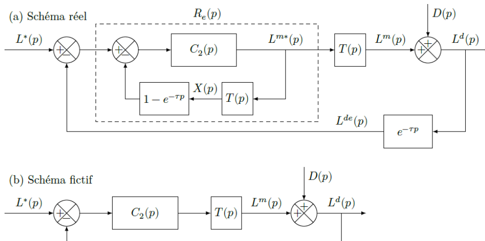
FIGURE 12.6 – Modèle de commande avec une boucle interne intégrée
