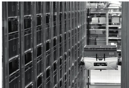
FIGURE 1.2 – Robot évoluant verticalement
