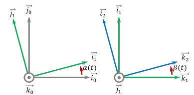
FIGURE 6.4 – Paramétrage
