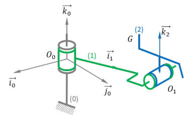
FIGURE 6.1 – Modélisation cinématique
