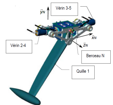
FIGURE 12.2 – Modèle volumique 3D
