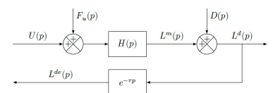
FIGURE 13.6 – Modèle du procédé pour la conception de la loi de commande de la chaîne d'asservissement
