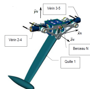
FIGURE 11.1 – Modèle volumique 3D
