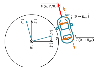
FIGURE 8.3 – Dérapiage
