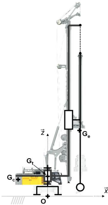
FIGURE 4.7 – Position des centres de gravité des différents solides.
