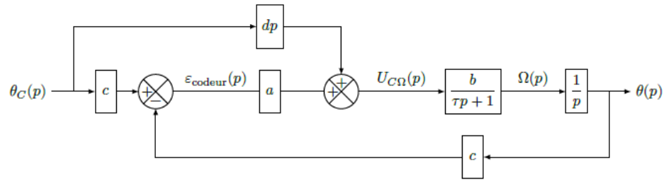
FIGURE 1.5 – Structure avec anticipation
