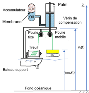
FIGURE 6 – Schéma d'implantation du PHV (non à l'échelle)
