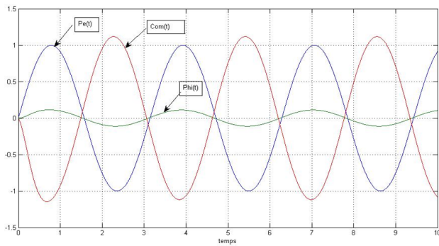
FIGURE 1.3 – Réponse de l'axe à une perturbation sinusoïdale
