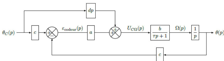
FIGURE 1.6 – Structure avec anticipation
