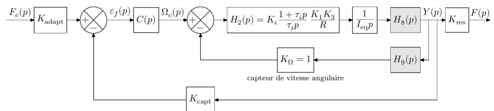
FIGURE 1.17 – Schéma-blocs de l'asservissement de la force développée par un actionneur linéaire
