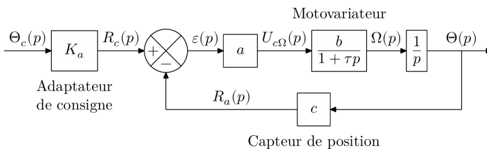
FIGURE 1.11 – Schéma-bloc de la commande en position du moteur
