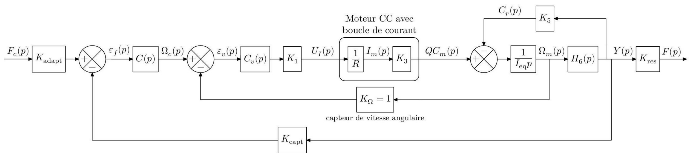
FIGURE 1.14 – Schéma-blocs de l'asservissement de force développée par un actionneur linéaire placé sur le banc d'essai
