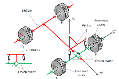
FIGURE 5.6 – Modèle du châssis
