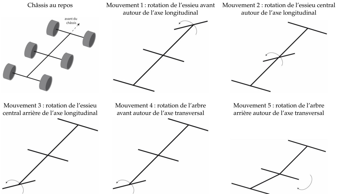
FIGURE 5.3 – Illustration des mouvements de déformation du châssis
