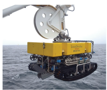
FIGURE 1.9 : ROV suspendu à la grue portique
