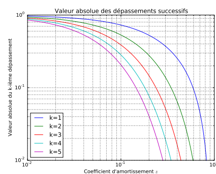
(b) Abaques des dépassements
