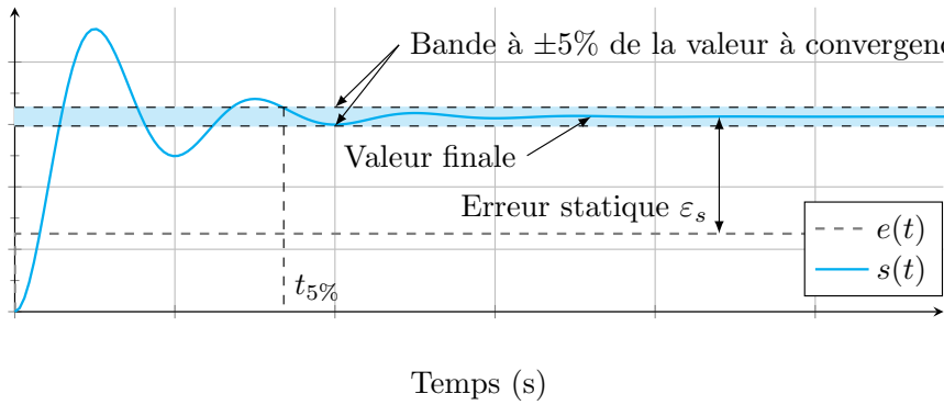
FIGURE 1.4 : Performances sur une réponse à un échelon.
