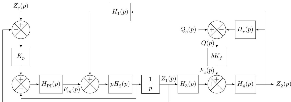
FIGURE 9 : Modèle de la chaîne d'asservissement complète
