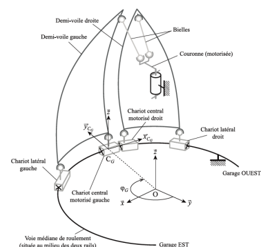
FIGURE 3.5 : Schéma d'architecture de la voile solaire
