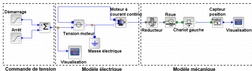
FIGURE 3.6 : Modèle multiphysique du déplacement d'une demi-voile
