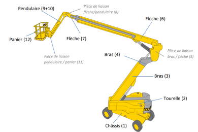
FIGURE 4.9 : Architecture globale de la nacelle
