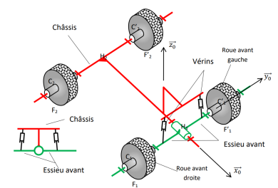
FIGURE 4.10 : Modèle du châssis
