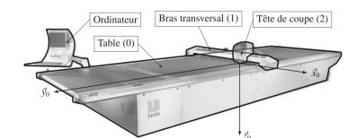
FIGURE 1.6 : Structure d'une table de découpe de tissus
