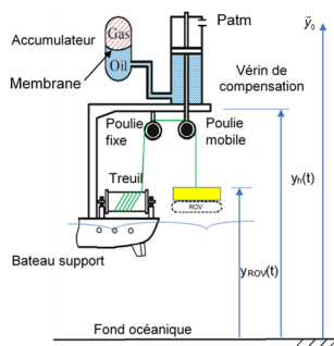
FIGURE 1.13 : Schéma d'implantation du PHV (non à l'échelle)
