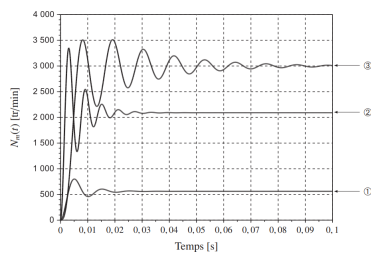
FIGURE 1.10 : Évolutions simulées de \omega_m(t) .
