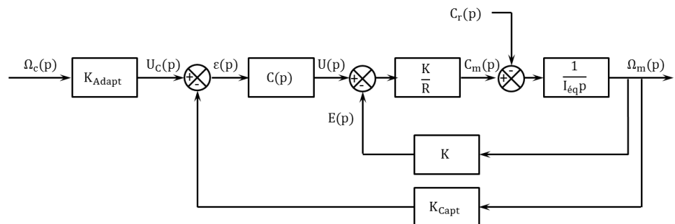
FIGURE 6 : Régulation en vitesse du banc d'essai.
