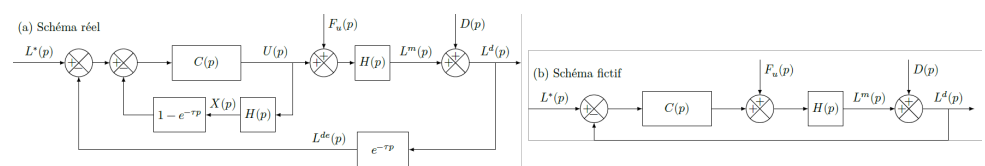
FIGURE 10 : Structure de commande adaptée aux systèmes à retard.
