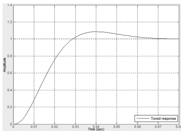
FIGURE 7 : Réponse temporelle système réglé.
