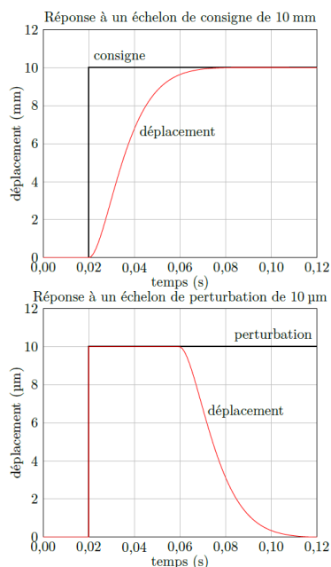
FIGURE 12 : Evolutions temporelles de la position L^d(t)
