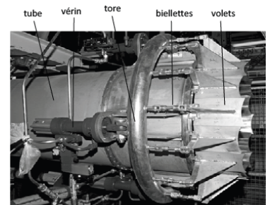
Tuyère à ouverture variable
