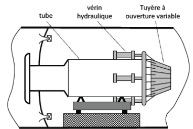
Document 3 – Réacteur simulé (compartment B)
