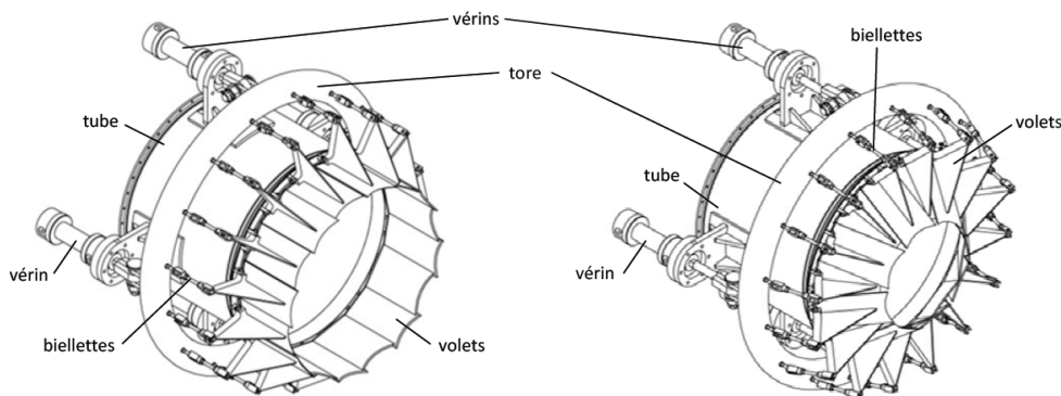
Document 4 – Tuyère ouverte
