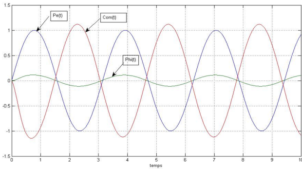
FIGURE 1.3 : Réponse de l'axe à une perturbation sinusoïdale
