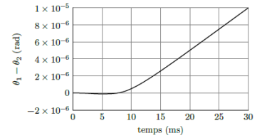
FIGURE 1.9 : \theta_1 - \theta_2 en fonction du temps
