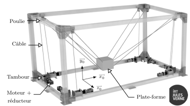
FIGURE 1.12 : Robot à câbles CAROCA
