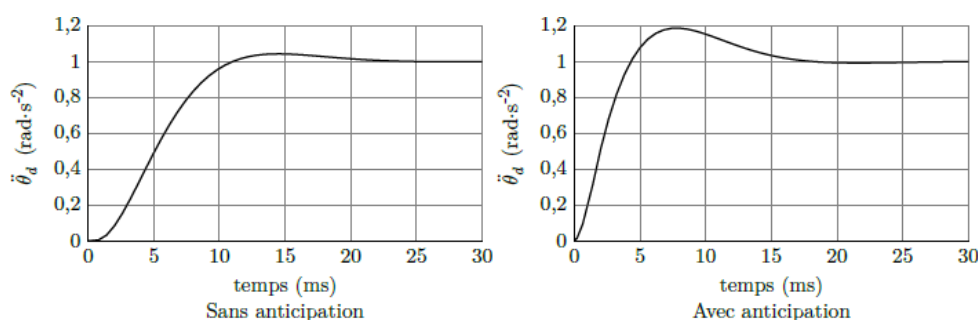
FIGURE 1.7 : Accélération du dossier avec et sans anticipation
