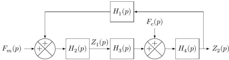
FIGURE 4 – Modèle de l'outil et porte-outil
