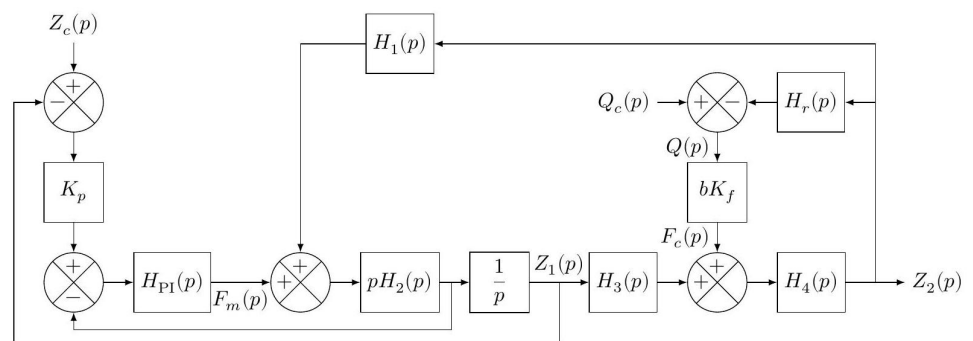
FIGURE 8 – Modèle de la chaîne d'asservissement complète
