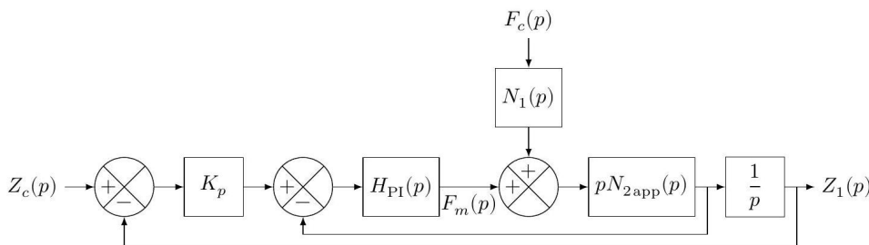
FIGURE 7 – Modèle de la régulation en position et en vitesse du porte-outil
