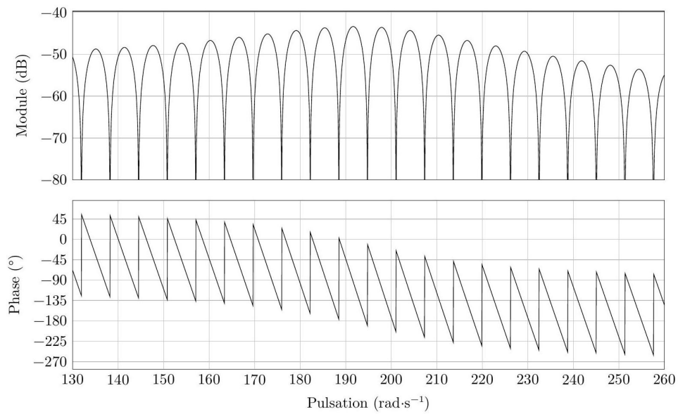
FIGURE 10 – Diagramme de Bode de la boucle ouverte du schéma bloc de la figure 9
