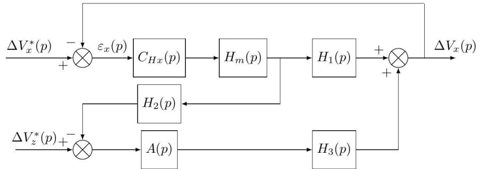
FIGURE 12 : Schéma-bloc intermédiaire
