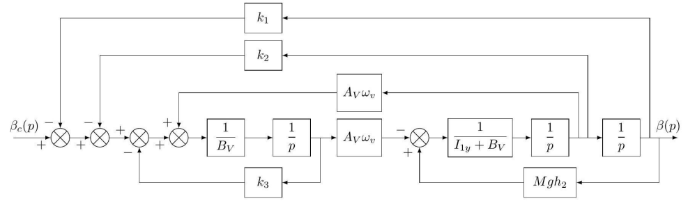
FIGURE 4 : Schéma-bloc de l'asservissement de l'angle de roulis \beta avec exploitation de trois mesures.
