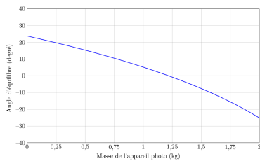
FIGURE 6.5 : Angle d'équilibre \alpha_0 en fonction de la masse de l'appareil photo m_4
