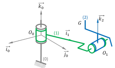
FIGURE 6.3 : Modélisation cinématique
