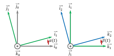
FIGURE 6.2 : Paramétrage
