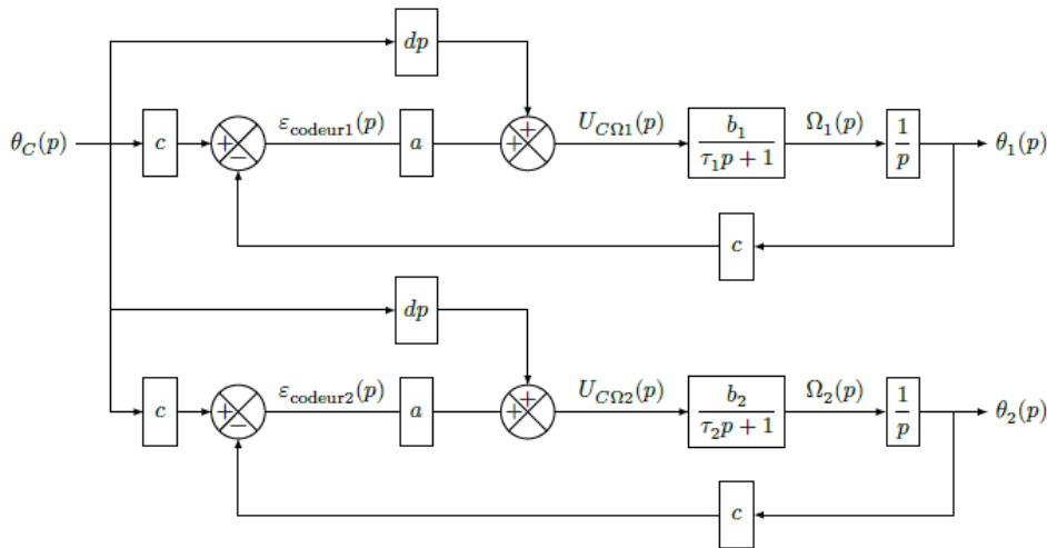
FIGURE 2.8 : Commande simultanée des deux moteurs
