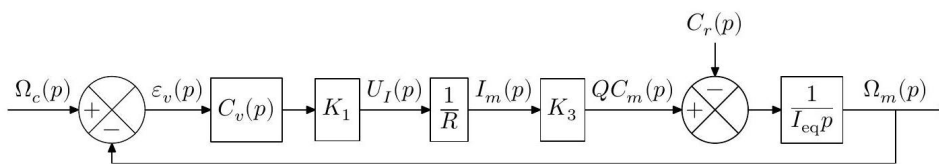
FIGURE 2.14 : Schéma-blocs de la boucle d'asservissement de la vitesse angulaire du moteur électrique
