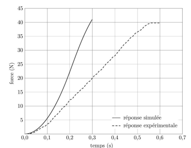
FIGURE 2.18 : Réponses temporelles du modèle et expérimentale, pour une consigne en échelon de force de 40 N
