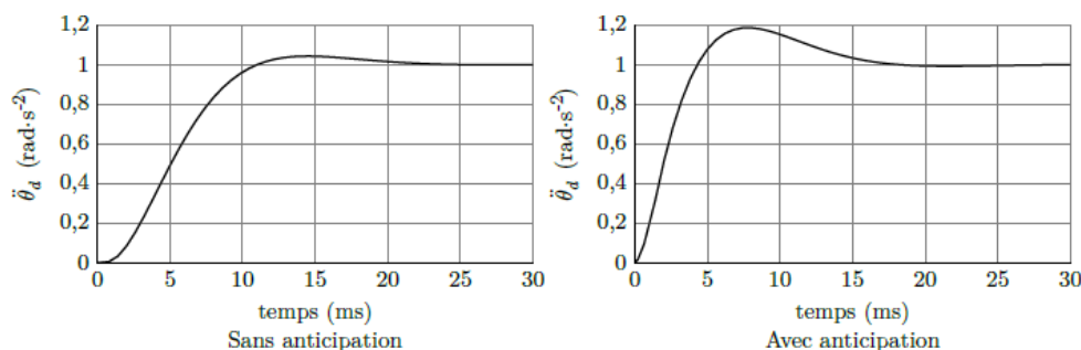
FIGURE 2.7 : Accélération du dossier avec et sans anticipation
