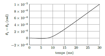
FIGURE 2.9 : \theta_1 - \theta_2 en fonction du temps
