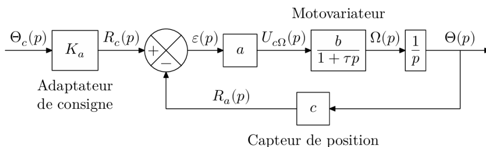
FIGURE 2.11 : Schéma-bloc de la commande en position du moteur
