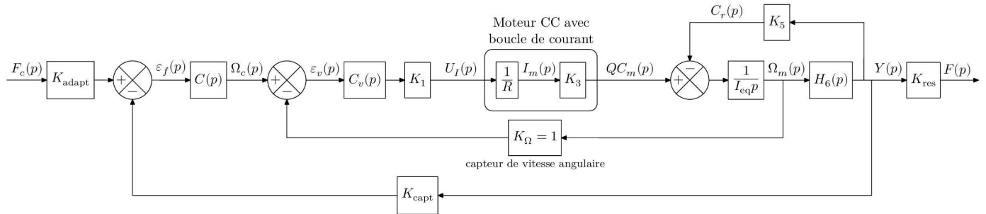
FIGURE 2.13 : Schéma-blocs de l'asservissement de force développée par un actionneur linéaire placé sur le banc d'essai
