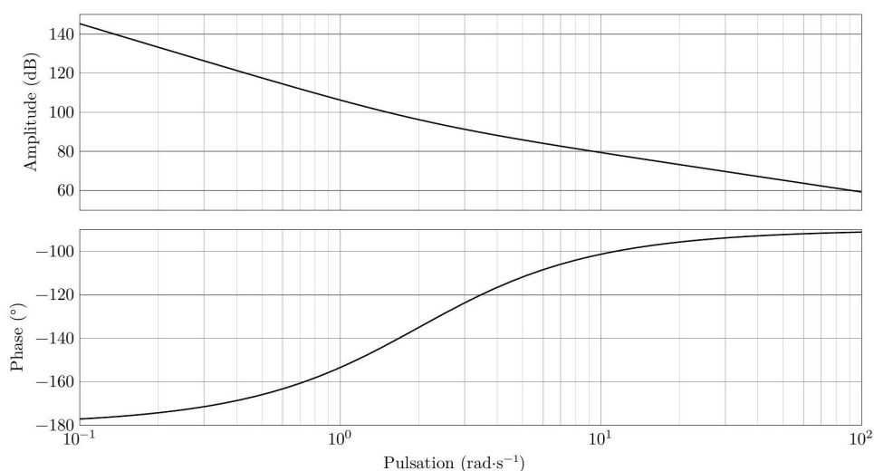
FIGURE 2.15 : Diagramme de Bode de H_{BOv}(p)
