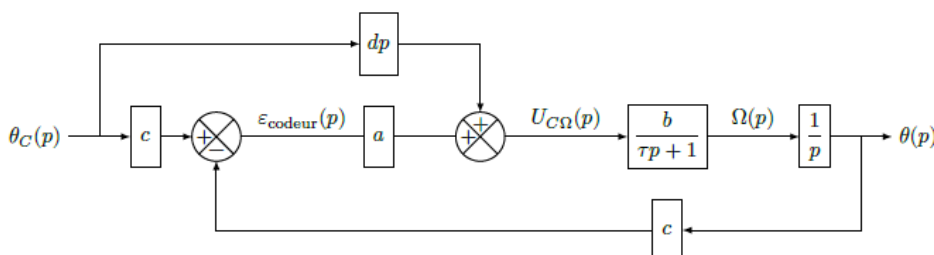
FIGURE 2.6 : Structure avec anticipation
