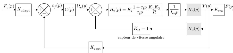
FIGURE 2.16 : Schéma-blocs de l'asservissement de la force développée par un actionneur linéaire
