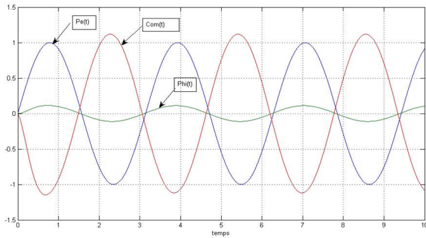
FIGURE 2.3 : Réponse de l'axe à une perturbation sinusoïdale
