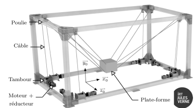
FIGURE 2.10 : Robot à câbles CAROCA
