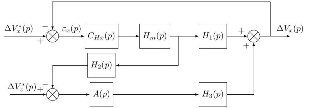
FIGURE 7 : Schéma-bloc intermédiaire
