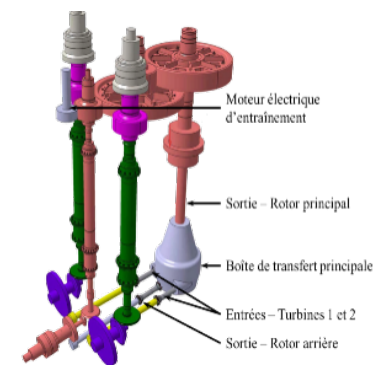
FIGURE 19 : Représentation de la BTP
