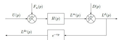
FIGURE 26 : Modèle du procédé pour la conception de la loi de commande de la chaîne d'asservissement
