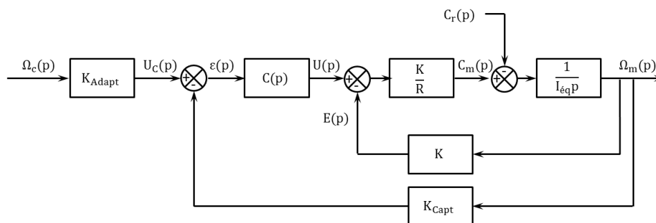
FIGURE 18 : Régulation en vitesse du banc d'essai.
