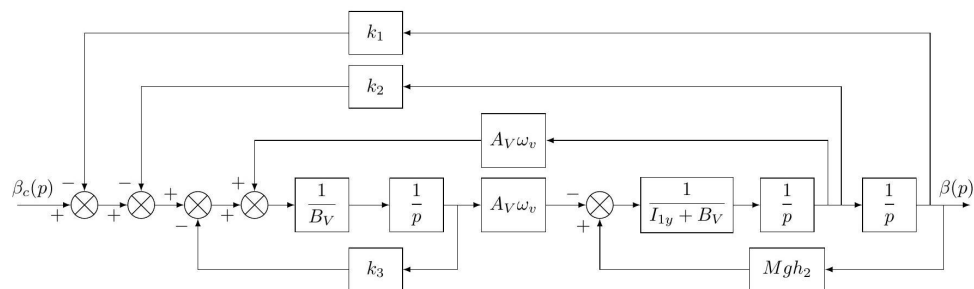
FIGURE 4 : Schéma-bloc de l'asservissement de l'angle de roulis \beta avec exploitation de trois mesures.
