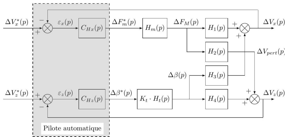
FIGURE 5 : Schéma-bloc couplé de l'asservissement des vitesses horizontale et verticale
