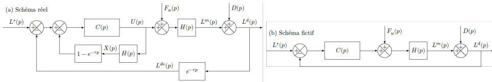
FIGURE 28 : Structure de commande adaptée aux systèmes à retard.
