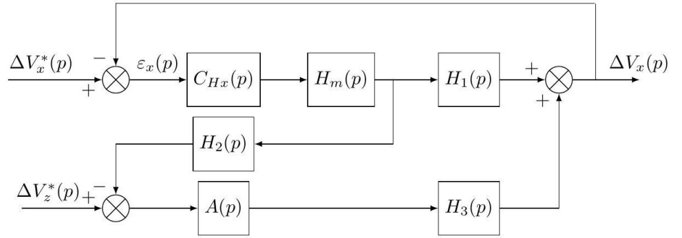
FIGURE 12 : Schéma-bloc intermédiaire
