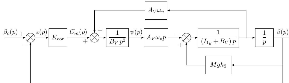
FIGURE 3 : Schéma bloc de l'asservissement de l'angle de roulis \beta avec un correcteur proportionnel.
