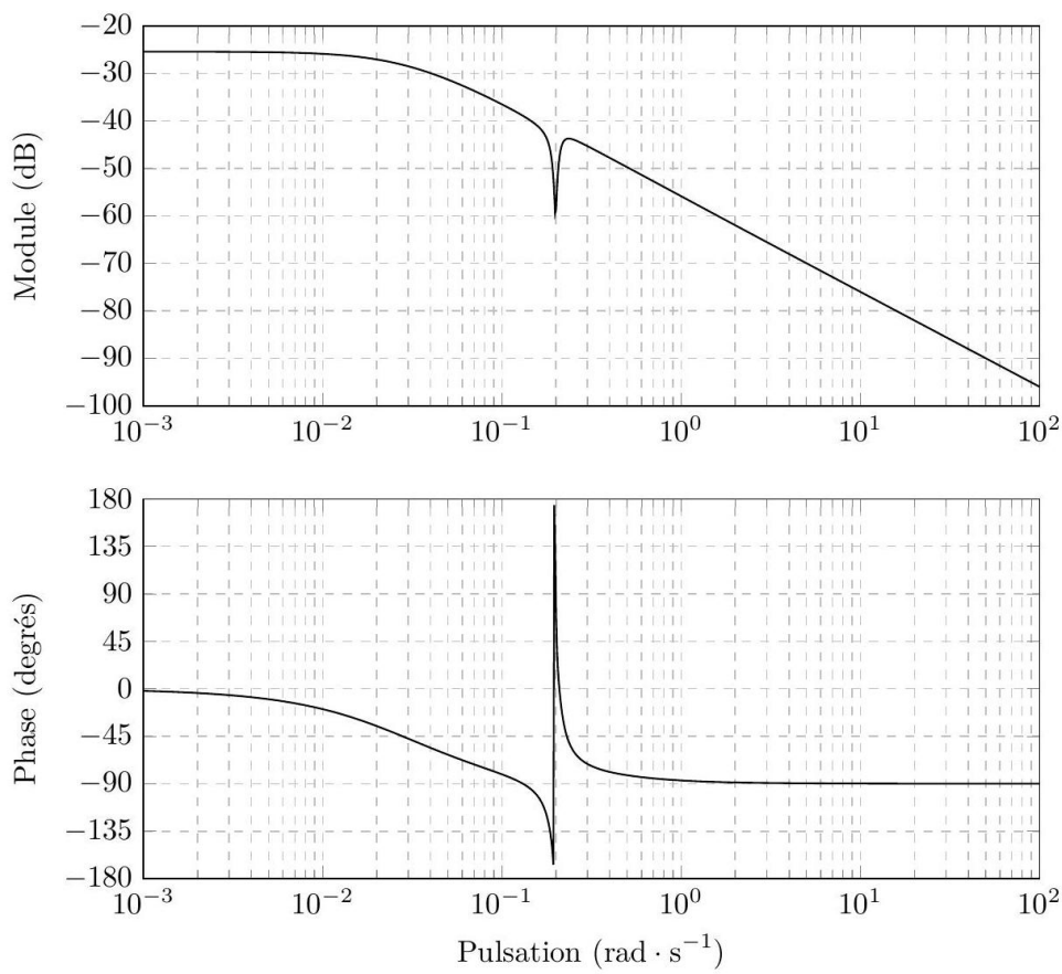
FIGURE 14 : Diagramme de Bode de H_1(p) - B(p)
