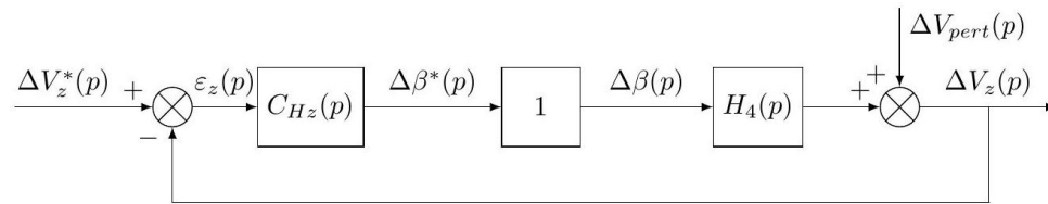
FIGURE 6 : Boucle de vitesse verticale linéarisée et découplée
