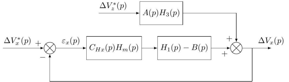
FIGURE 13 : Boucle de vitesse horizontale perturbée
