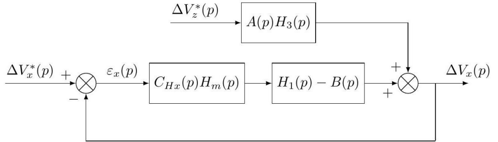
FIGURE 8 : Boucle de vitesse horizontale perturbée
