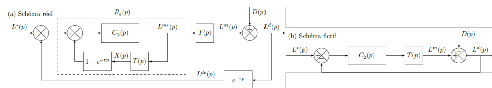
FIGURE 29 : Modèle de commande avec une boucle interne intégrée
