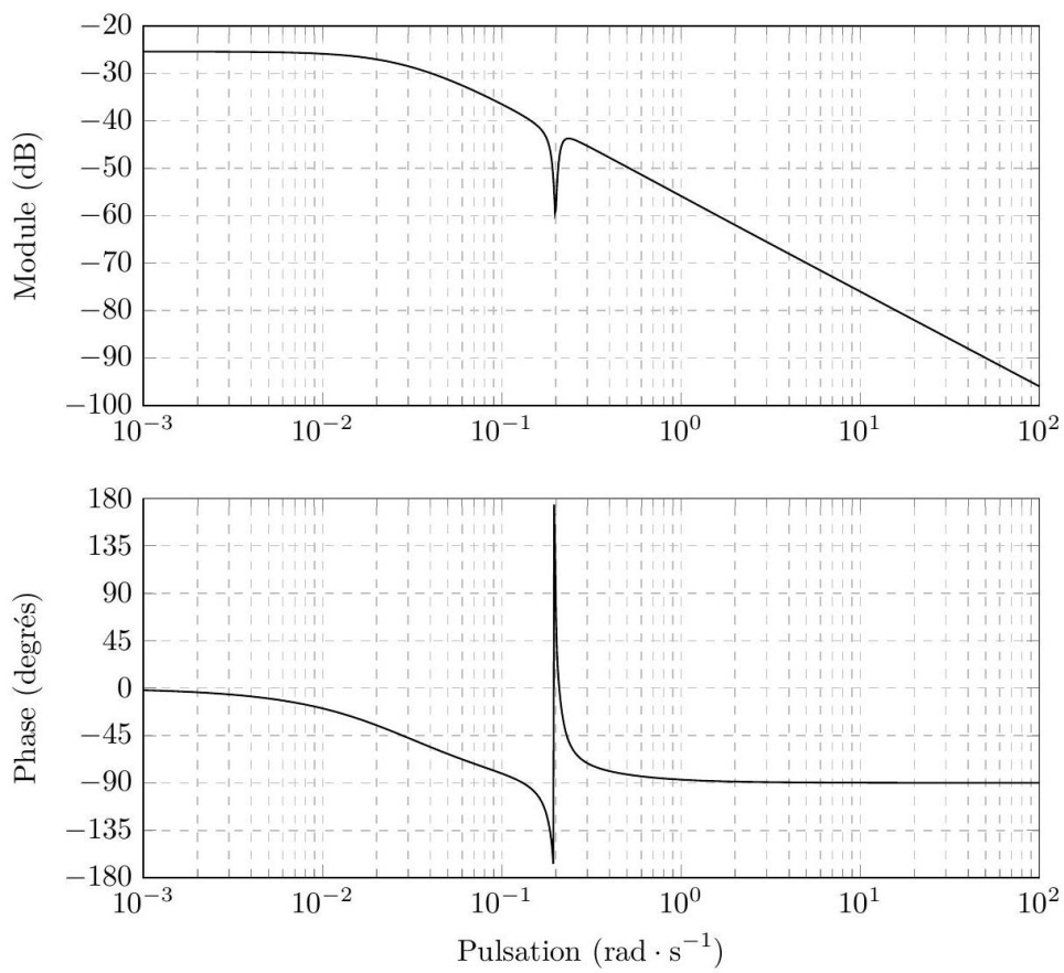
FIGURE 9 : Diagramme de Bode de H_1(p) - B(p)
