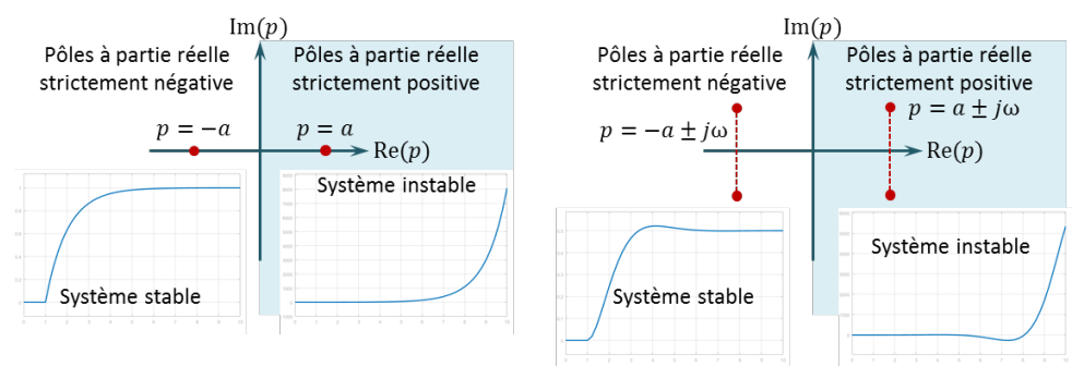
FIGURE 2.1 : Représentation d'un système à pôle simple et à pôles conjugués dans le plan complexe – Réponse indicelle
