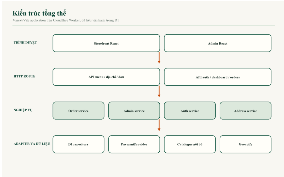
Hình 4.1. Kiến trúc tổng thể
