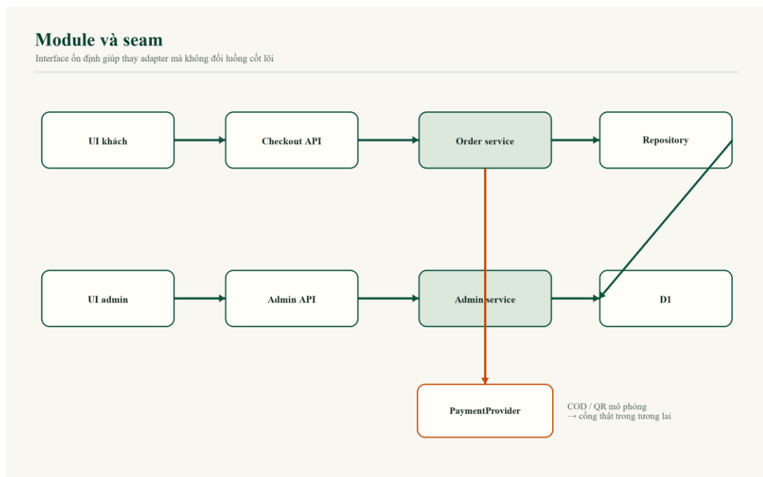
Hình 4.2. Sơ đồ module và các seam chính
