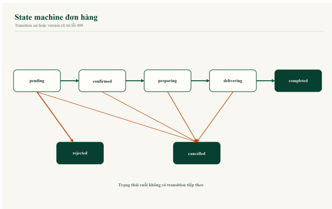
Hình 4.5. State machine xử lý đơn
