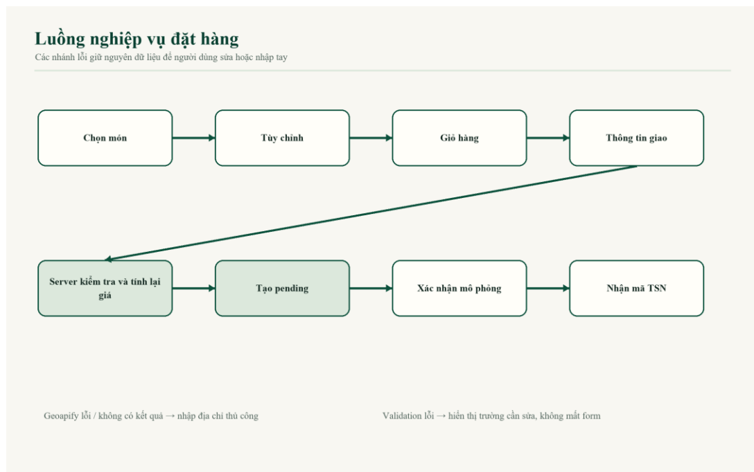
Hình 3.2. Luồng nghiệp vụ đặt hàng
