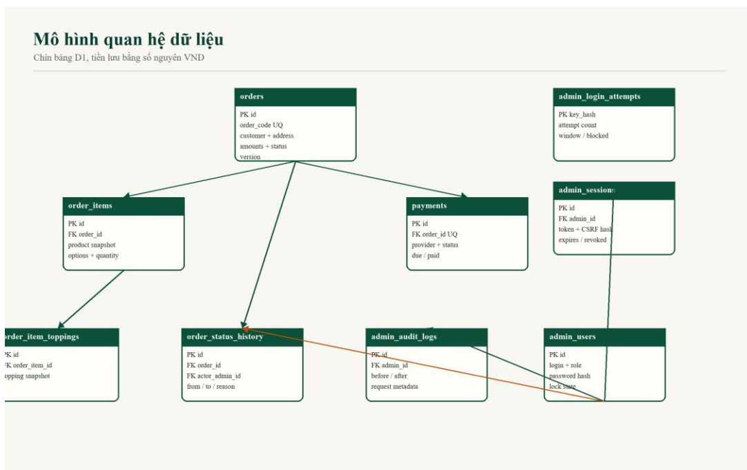
Hình 4.4. Mô hình quan hệ dữ liệu D1
