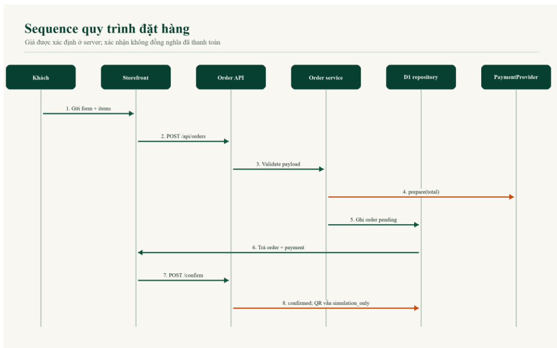
Hình 4.3. Sequence quy trình đặt hàng
