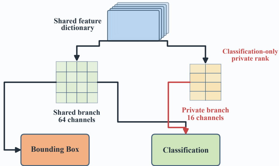
(b) SRPA-YOLO
