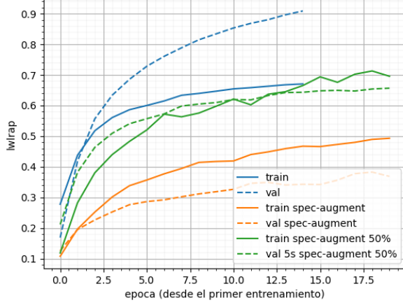
Figura 8: LwLrap de entrenamiento para modelo basado en MobileNet regularizado, utilizando SpecAugment y luego reduciendo su aplicación al 50 % de las muestras.
